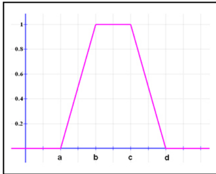
Figura 1. Función rectangular
